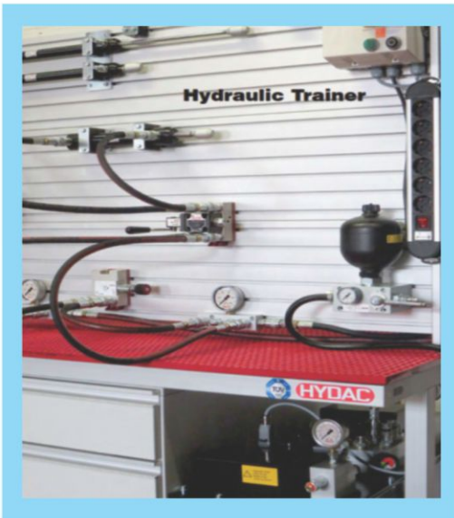
HYDRAULIC TRAINER
